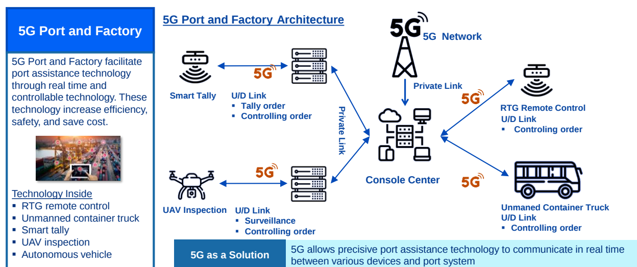
รูปที่ 7-11: สถาปัตยกรรมพื้นฐาน 5G ของท่าเรืออัจฉริยะ 5G
